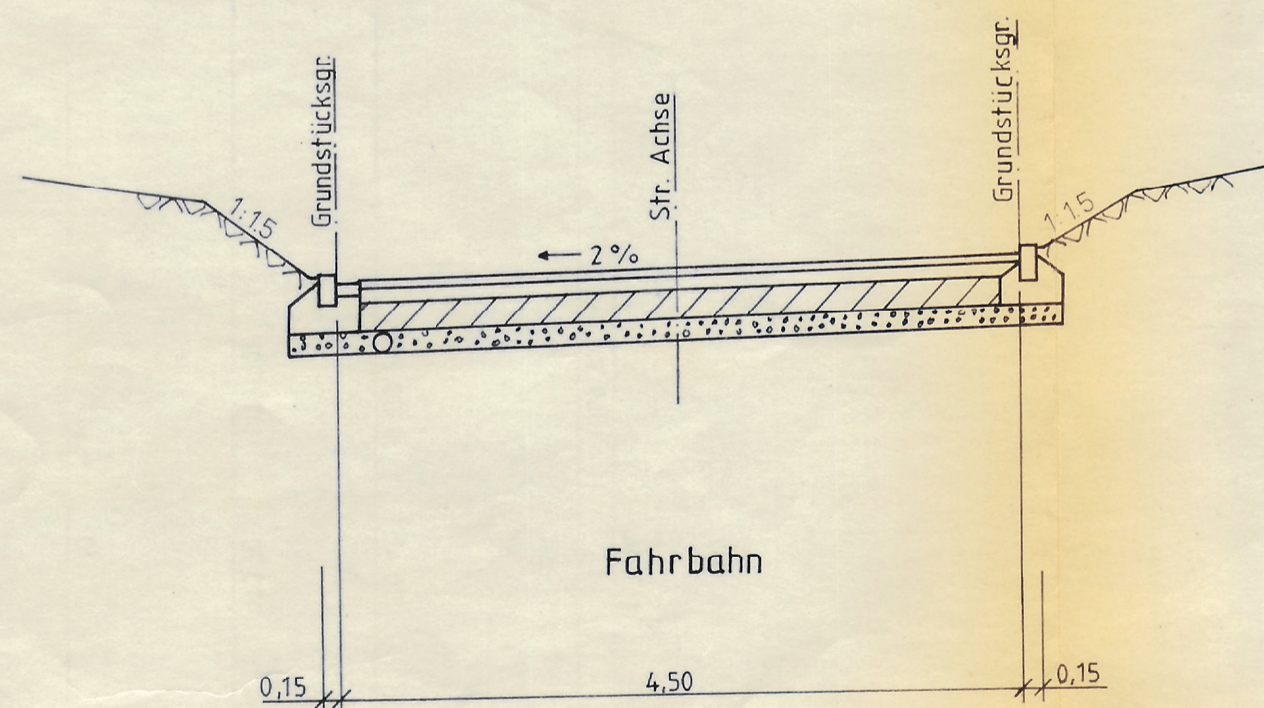
Regelschnitt Wohnstraße
