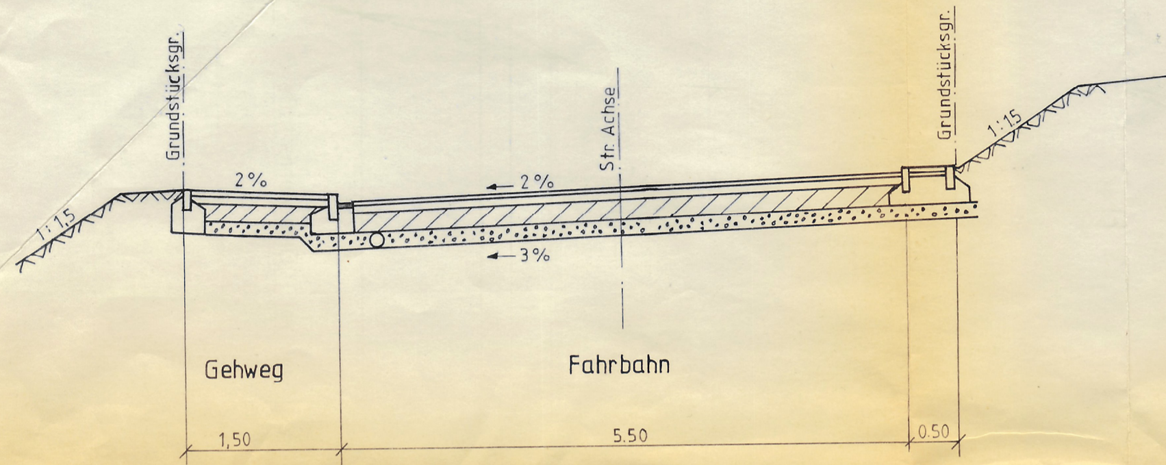
Regelschnitt Haupterschließungsstraße A
