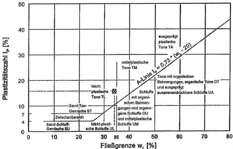
Plastizitätsdiagramm
